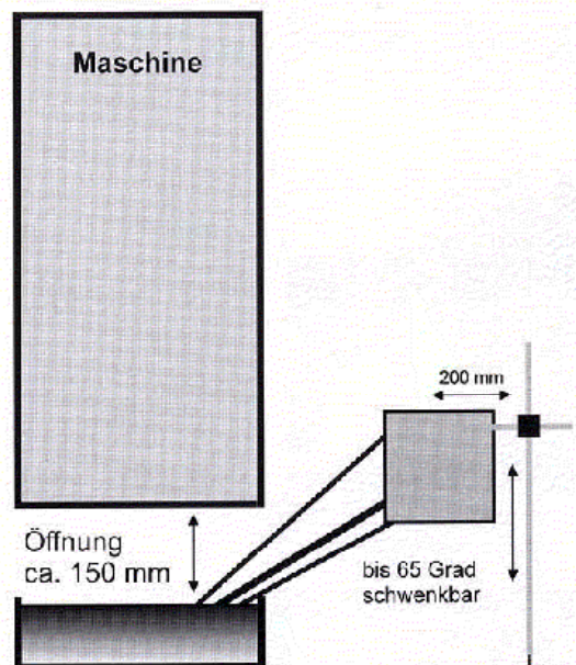
Behälter nur seitlich zugänglich
