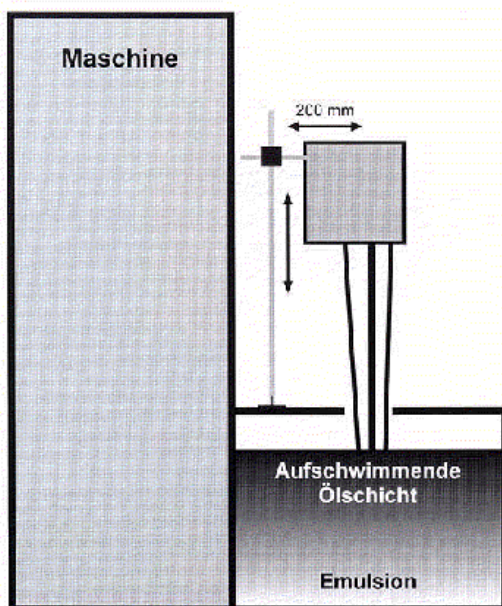
Behälter von oben zugänglich
